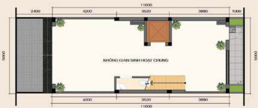
MẶT BẰNG TẦNG 1
