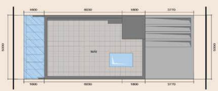
MẶT BẰNG MÁI
