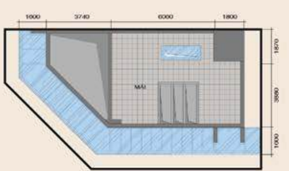
MẶT BẰNG MÁI
