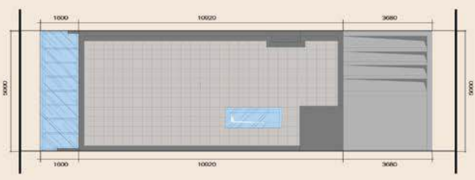
MẶT BẰNG MÁI
